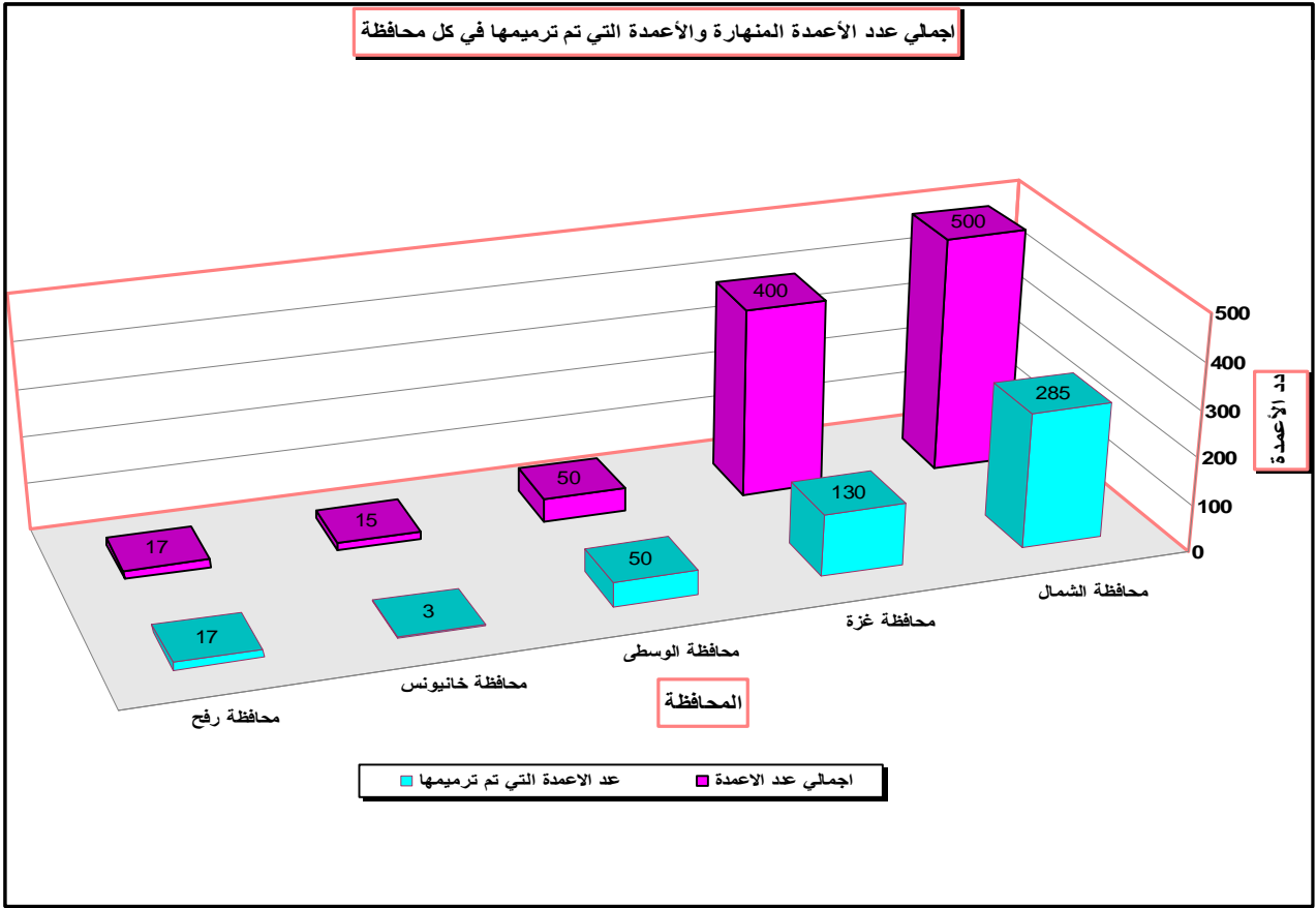
شكل رقم (١) يوضح مناطق العمل وإجمالي عدد الأعمدة المنهارة والأعمدة التي تم ترميمها
